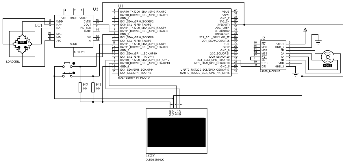
Fig. 5 Diagrama electrónico.
