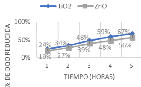
Fig. 5. Porcentaje de reducción de DQO en cada tratamiento.
