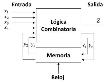
Fig. 1. Modelo de circuito secuencial síncrono.
